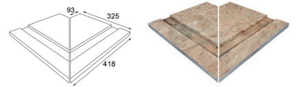
Esq. ext. borde desbordante Overflowing external edge 903878 Gris / 903888 Marrón / 903898 Mix JG760
