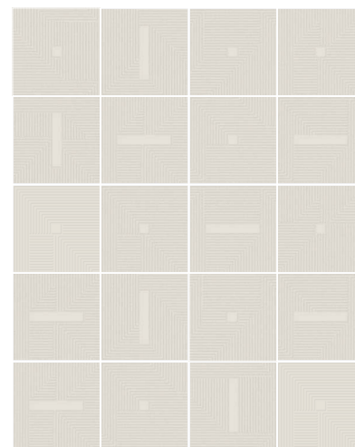
(1) Ronna G.258
