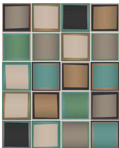
(1) Tauon G.285
